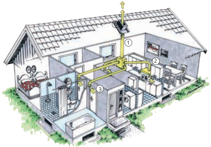
Exempel med frånluftsfläkt ① placerad på vind med frånluft från kök ②, badrum ③ och toalett ④. Frånluften förs till takhuv ⑤ över tak.
