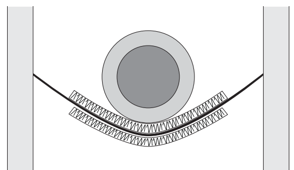
Innebygd kanal. Tilleggisolering av patentband med cellegummi.
